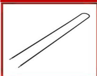
ТЭН-170АРозмер 8,5/Вать 0,4SВольт 230_000.180 Нержавик
