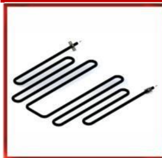
ТЭН Ватт 2,5 кВт,Вольт 230 Вт для тепловентилятора арт.001.050 Нержавик
