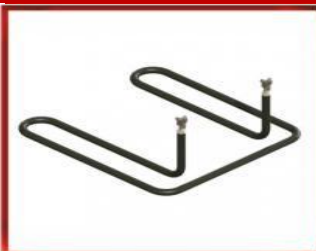
ТЭН 150-Розмер 7-8,5/ Вать1,4 кВтВольт 230_000.192-03 Нержавик
